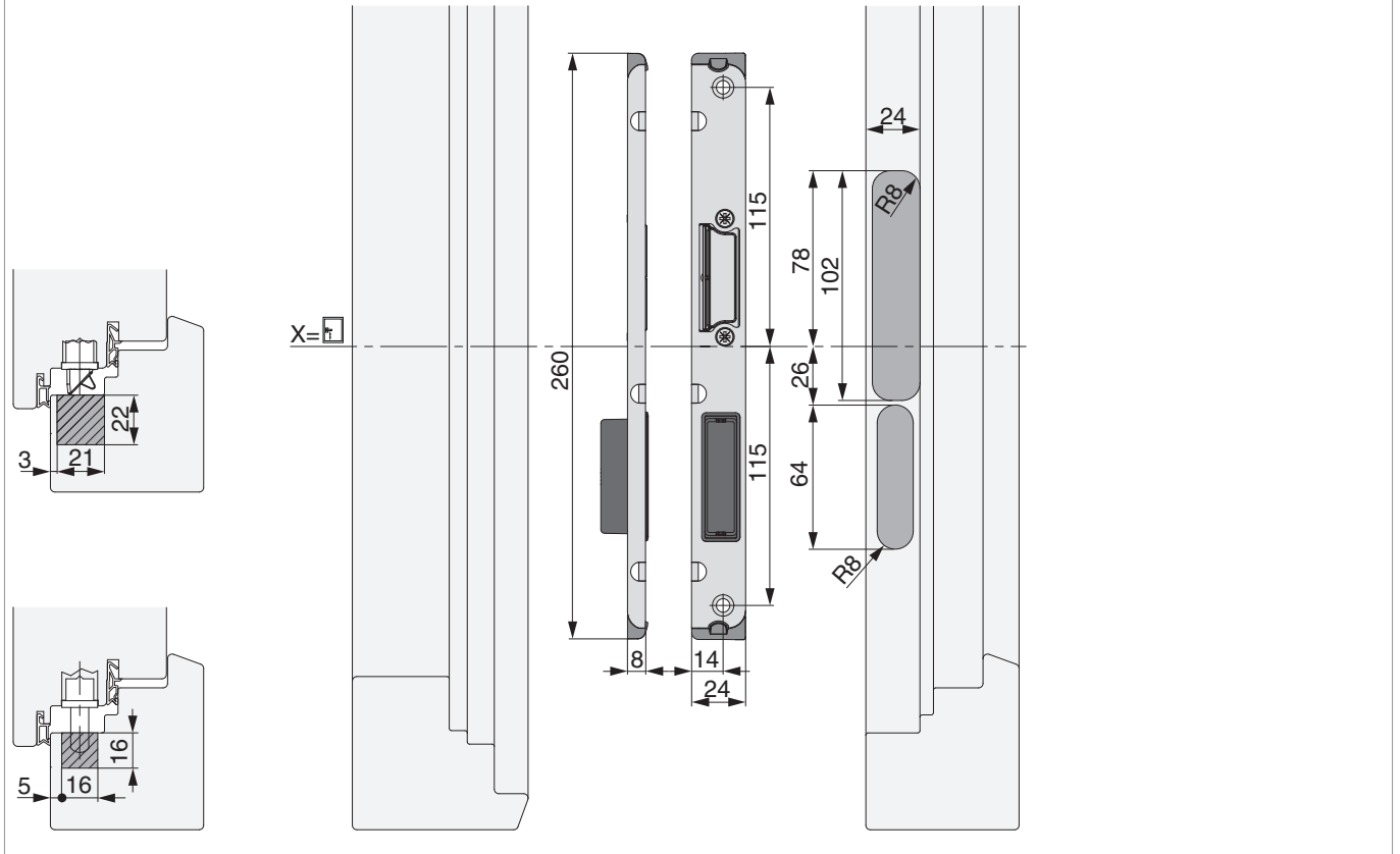
Fallen- und Riegel-Winkelschließblech
