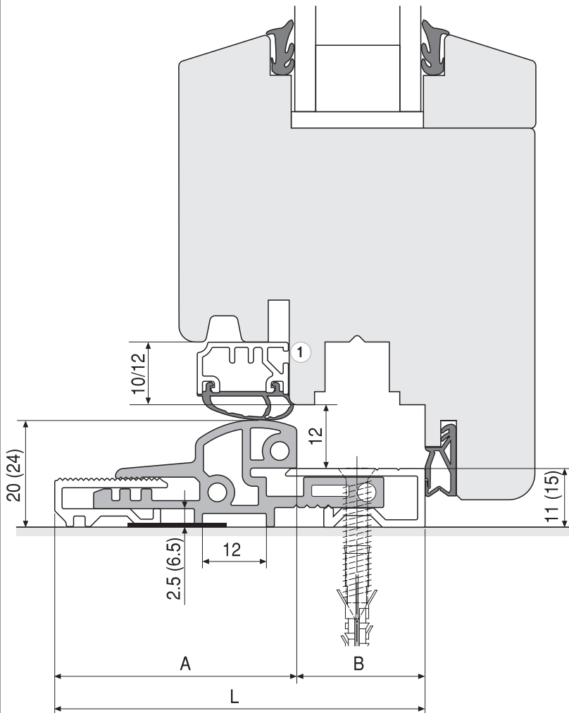
Schnitt Flügel
