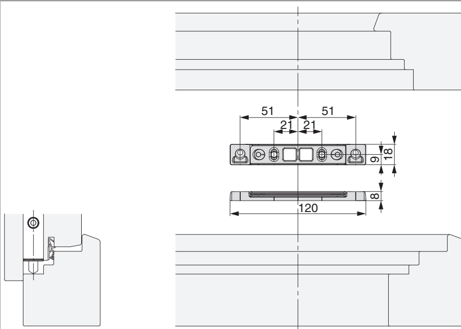
Riegelschließteile
