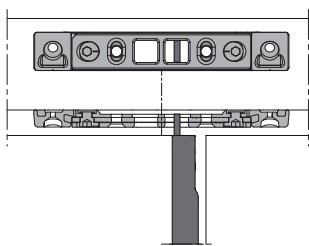
2-Flg. Tür mit 1 Riegel
