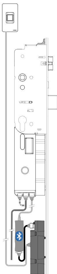
Möglichkeit 2: Anschluss zwischen openDoor Zutritts- kontrolle und Motor
