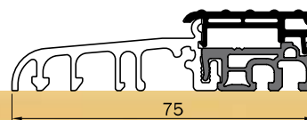
BKV 75 TB
