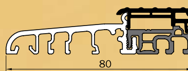
BKV 80 TB
