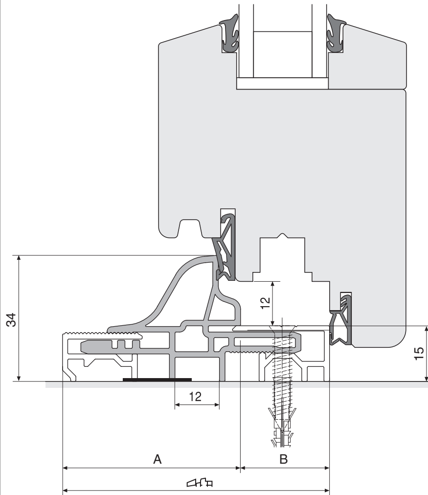
Schnitt Flügel
